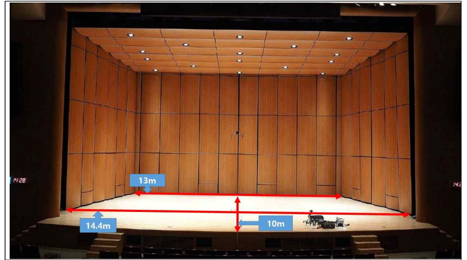
◎ 음향반사판 및 장치반입구 사진(수치 표시)
